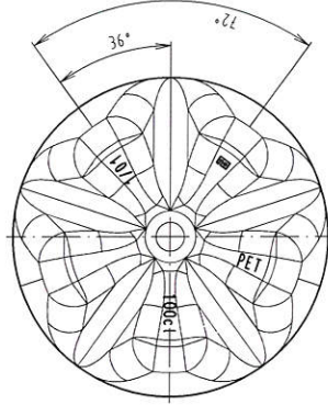
Bodenansicht M1:1
